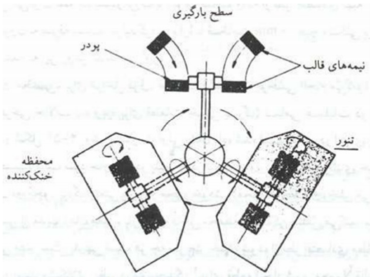
شکل ( 1 ) : عملیات قالب گیری دورانی
